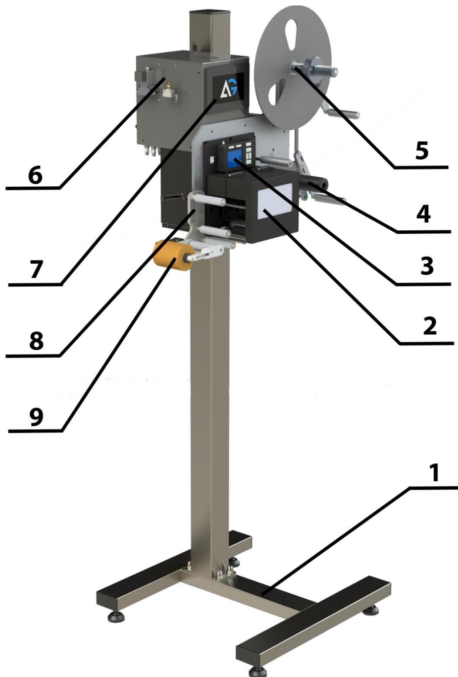
Рисунок. Внешний вид и обозначение основных узлов принтера-аппликатора этикеток Н-ПР-08.
