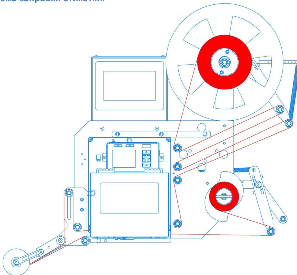
Рисунок. Схема заправки принтера-аппликатора Н-ПР-08.
