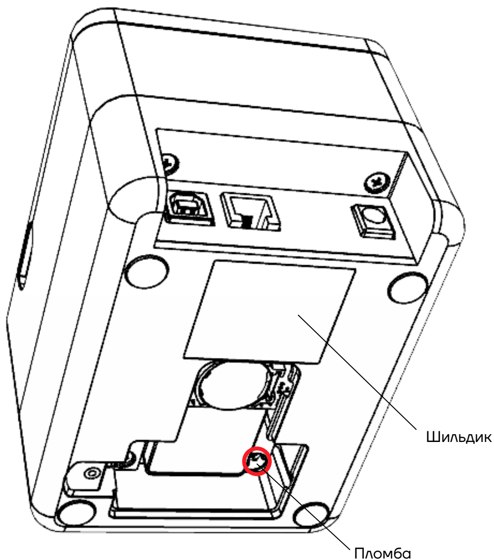
Рисунок 1. Расположение маркировки на корпусе ККТ (крышка отсека для ФН условно не показана)
