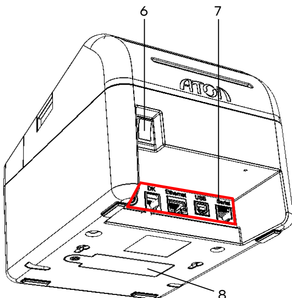
Рисунок 2. Вид снизу/сзади/слева
