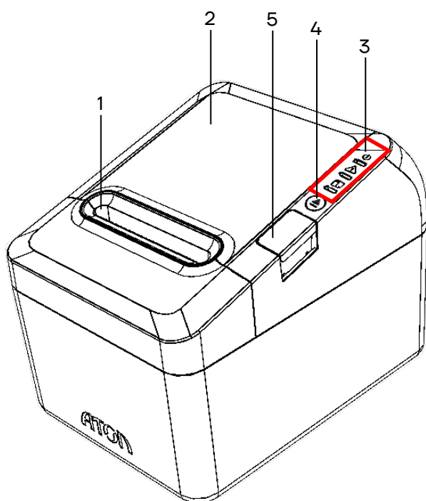
Рисунок 1. Вид сверху/сбоку/справа
