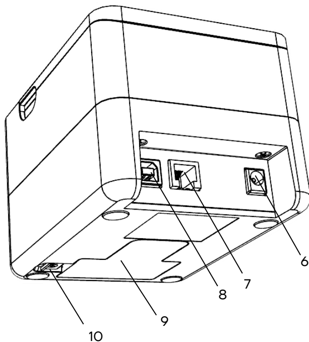
Рисунок 2. Вид сзади/сбоку/справа
