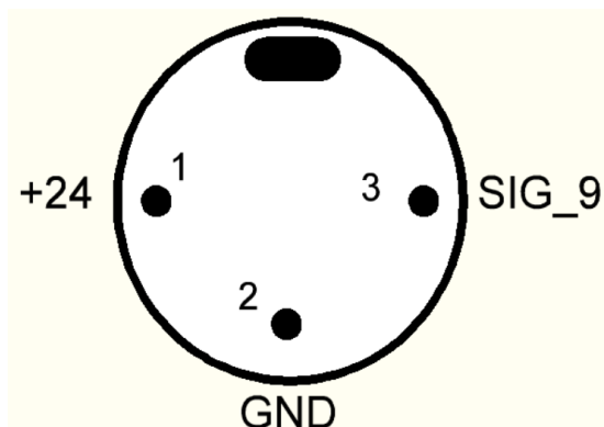
Рисунок. Схема распайки кабеля датчика окончания этикетки (разъем X5, GX-12-3pin).
