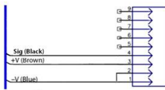
Рисунок. Схема распайки кабеля от датчика этикетки типа PNP. Разъем X3, DB-9.
