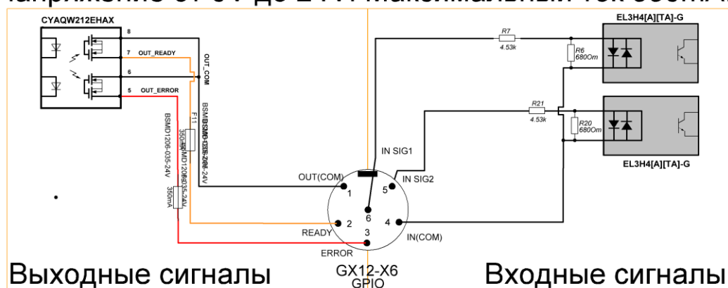
Рисунок. Схема распайки кабеля подключения внешних сигналов (разъем X6, GX-12-6pin).
