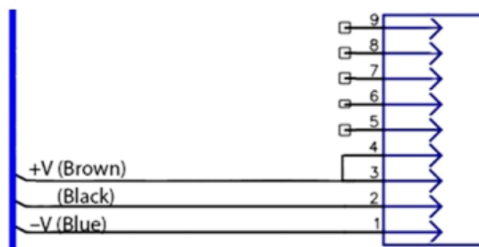
Рисунок. Схема распайки кабеля от датчика этикетки NPN. Разъем X3, DB-9.
