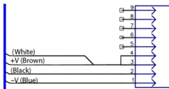
Рисунок. Схема распайки кабеля от датчика продукта типа NPN. Разъем X2, DB-9.
