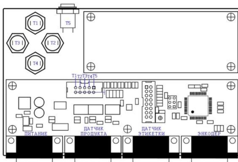
Рисунок. Обозначение разъемов контроллера.
