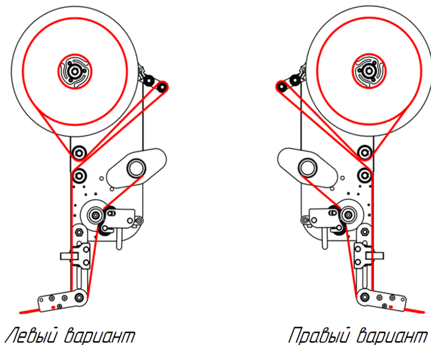
Рисунок. Схема заправки аппликатора А-150.
