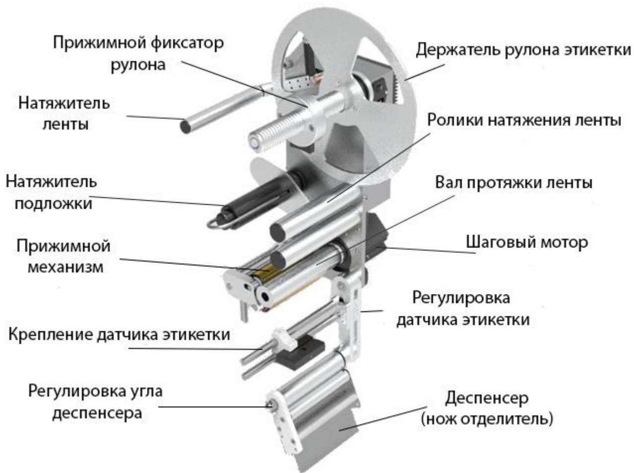
Рисунок. Внешний вид и обозначение основных узлов аппликатора этикеток А-150.
