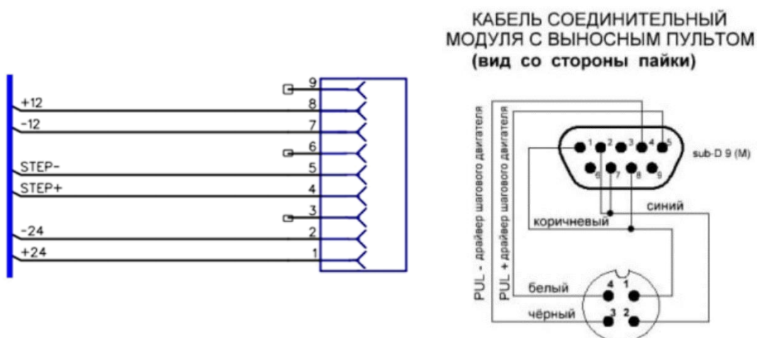
Рисунок. Схема распайки кабеля питания X1.
