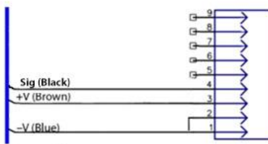
Рисунок. Схема распайки кабеля от датчика продукта типа PNP. Разъем X2, DB-9.
