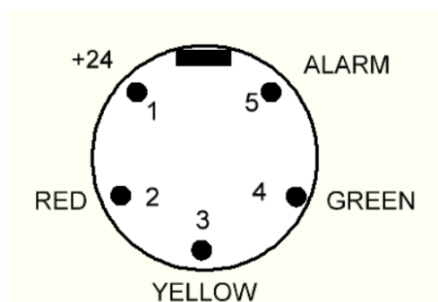
Рисунок. Схема распайки кабеля светофора (разъем X8, GX-12-5pin).
