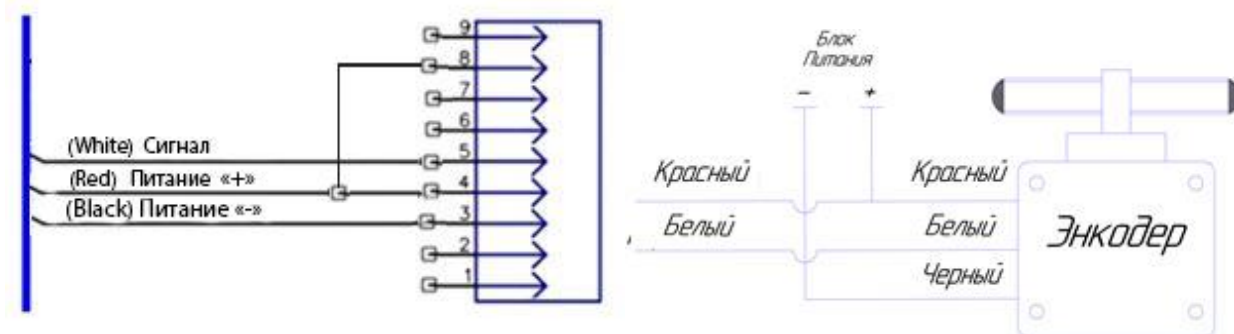
Рисунок. Схема распайки кабеля энкодера, запитанного от контроллера аппликатора.
