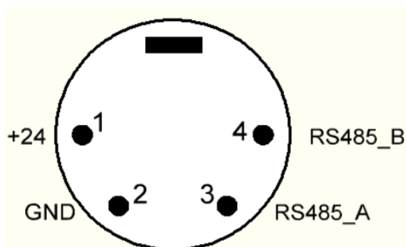
Рисунок. Схема распайки кабеля подключения тандема (разъем X7, GX-12-4pin).
