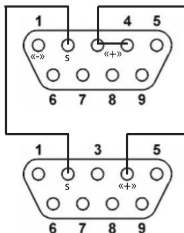
Рисунок. Схема распайки кабеля датчика продукта на два контроллера. Разъем X2, DB-9.
